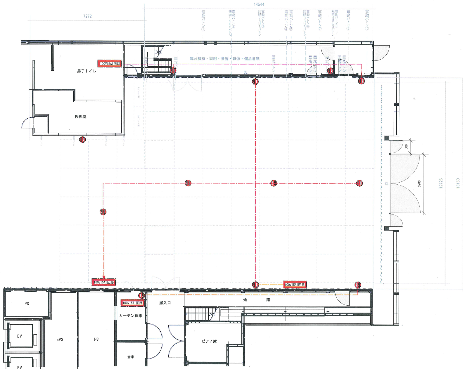
信毎メディアガーデン1Fホール 壁・床コンセント回路図【A3-1/100】
